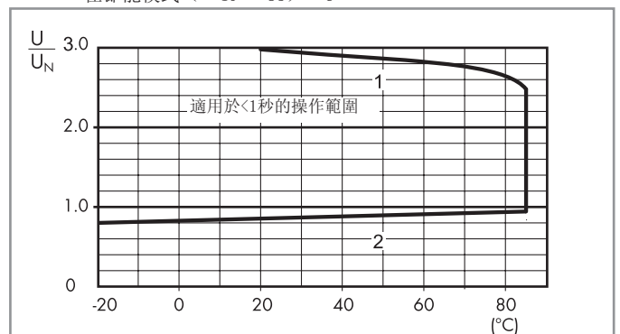
R 67 - 操作範圍與環境溫度, 67. xx-4300/4500 在節能模式 (-40...+85) ° C
