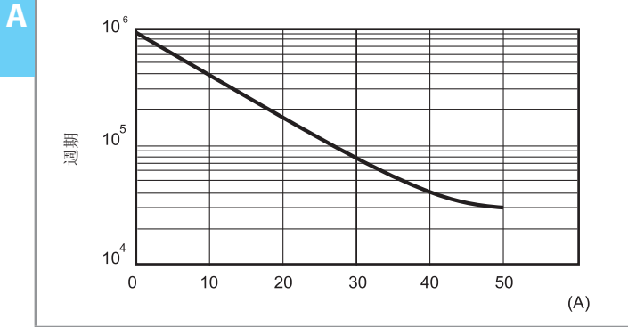
H 67 - 最大DC斷流容量 (67.xx-4300)
