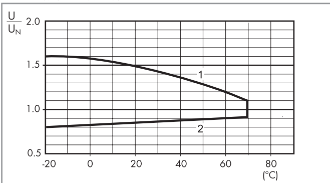
R 67 - 操作範圍與環境溫度, 67. xx-x300 標準 (連續) 線圈通電 (-40...+70) ° C
