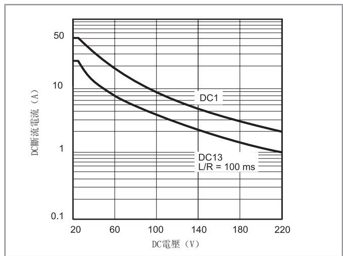
H 67 - 最大DC斷流容量 (67.xx-4500)
