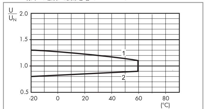
R 67 - 操作範圍與環境溫度, 67. xx-x500 標準 (連續) 線圈通電 (-40...+60) ° C
