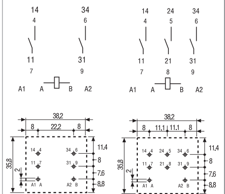
62.22 - 0300 铜触点侧视图
