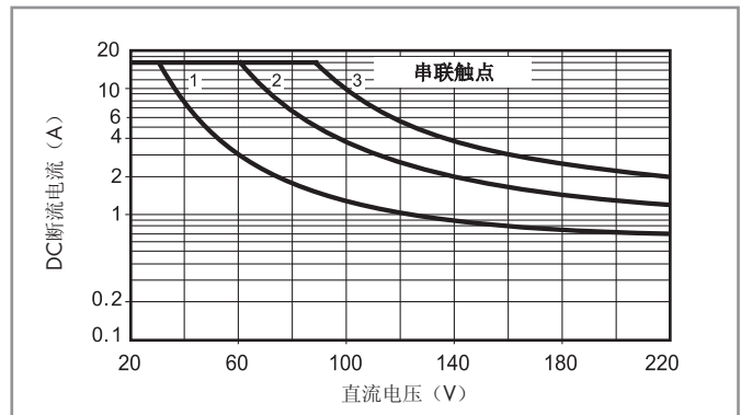
H 62 - 最大DC1断流容量 常开触点
