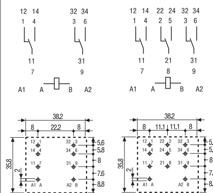
62.22 铜触点侧视图
