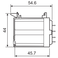
带有继电器的 062.08
